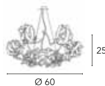
Gomitoli 3011/L8L 8 x max 60W G9 230V
