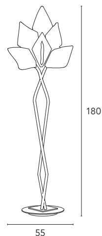
Alaska 2552/P6L 6 x max 40W G9 230V CE F
