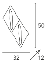
Alaska 2552/A2L 2 x max 40W G9 230V CE F
