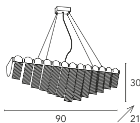
Lucidum 1310/S90R 8 x 60W E14 230V
