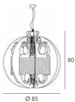
Sphera 2112/S6 6 x max 60W E14 230V
