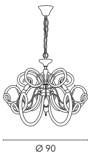
Vanity 1806/L12L 12 x max 60W E14 230V
