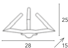
Stark 3030/A3L 3 x max 40W G9 230V ☼ CE V □
