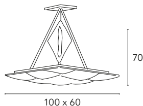
Alaska 2552/L10L 10 x max 40W G9 230V CE F
