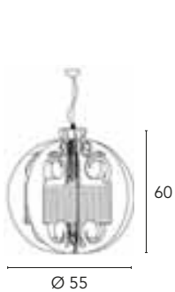
Sphera 2112/S 1 x max 100W E27 230V
