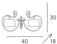
Romantica 3016/A2L 2x max 60W E14 230V ⚡ CE V □ ⊕
