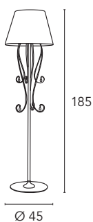
Romantica 3016/P 1x max 250W E27 230V ⚡ CE V □ ⊕
