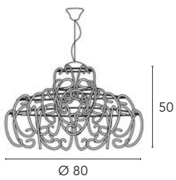
Gemini 2110/L9L 9 x max 60W G9 230V CE V
